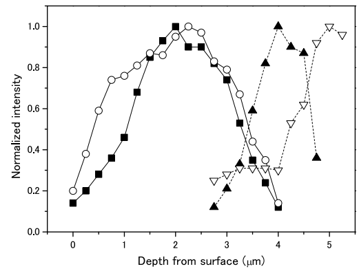
(d) OD-630°C-20min
